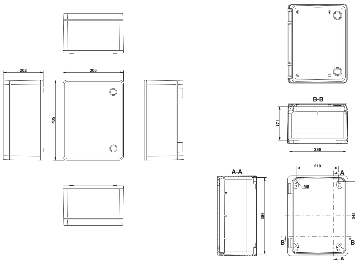
Esquema de dimensiones
