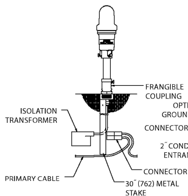
Stake Mounted ERL
