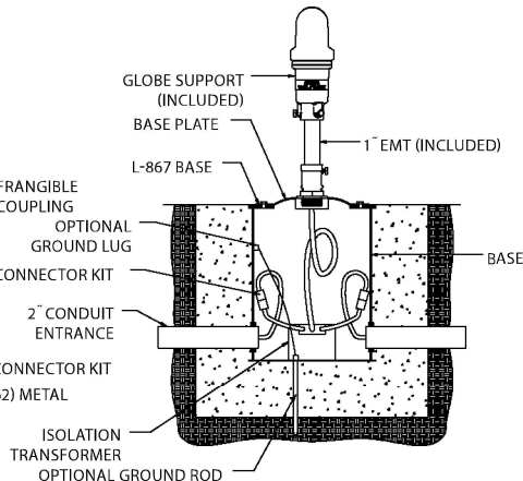
Base Mounted ERL
