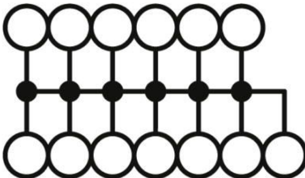
Diagrama eléctrico
