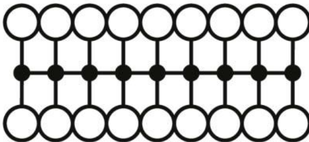
Diagrama eléctrico
