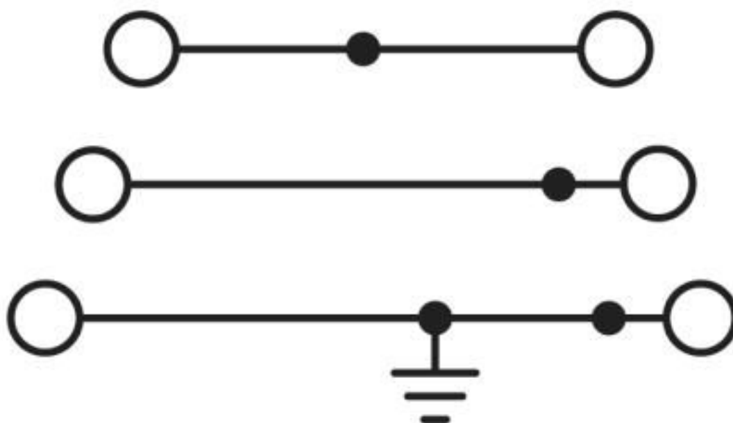
Diagrama eléctrico
