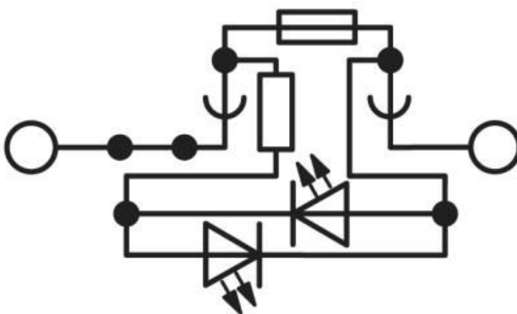
Diagrama eléctrico
