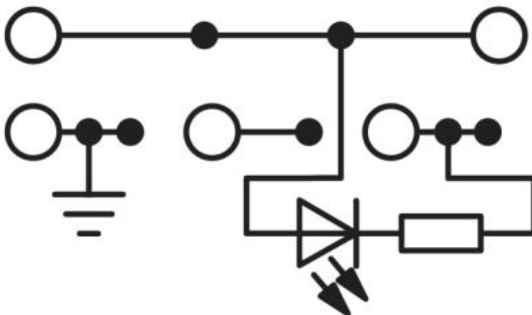
Diagrama eléctrico
