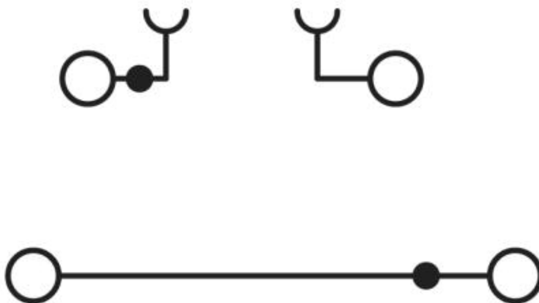
Diagrama eléctrico
