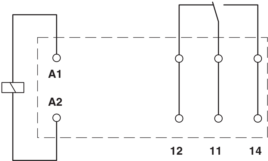
Diagrama eléctrico
