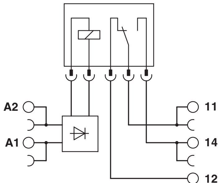
Diagrama eléctrico
