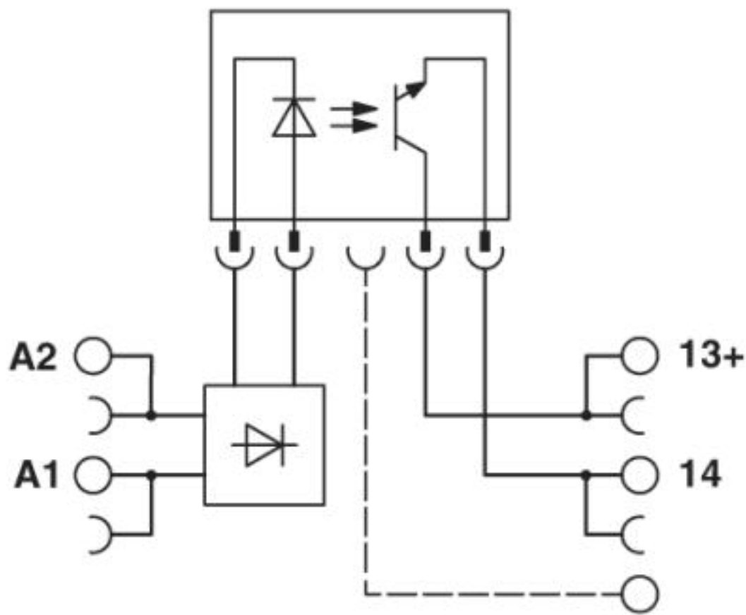
Diagrama eléctrico
