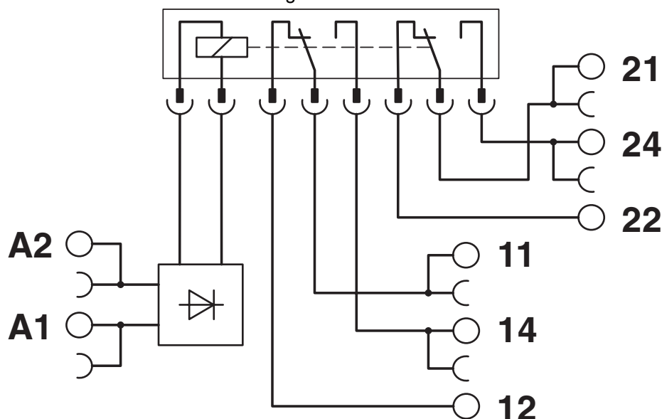
Diagrama eléctrico
