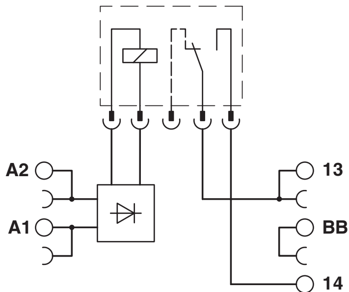
Diagrama eléctrico
