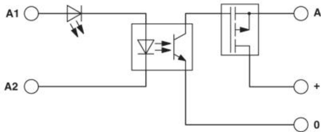
Diagrama eléctrico
