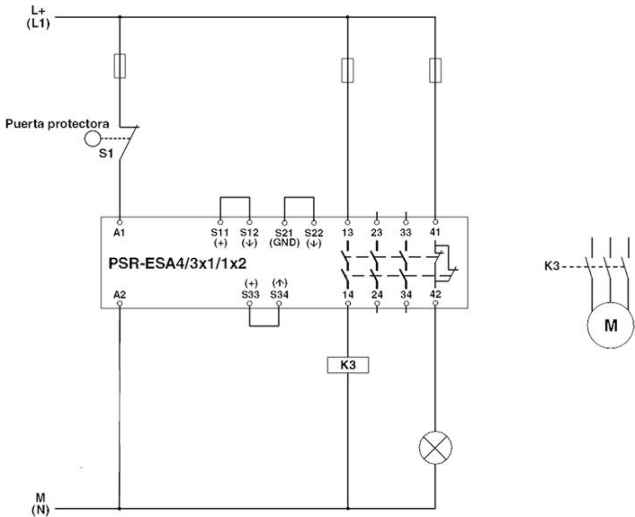
Diagrama eléctrico
