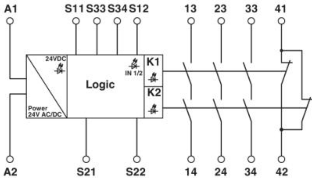
Diagrama eléctrico
