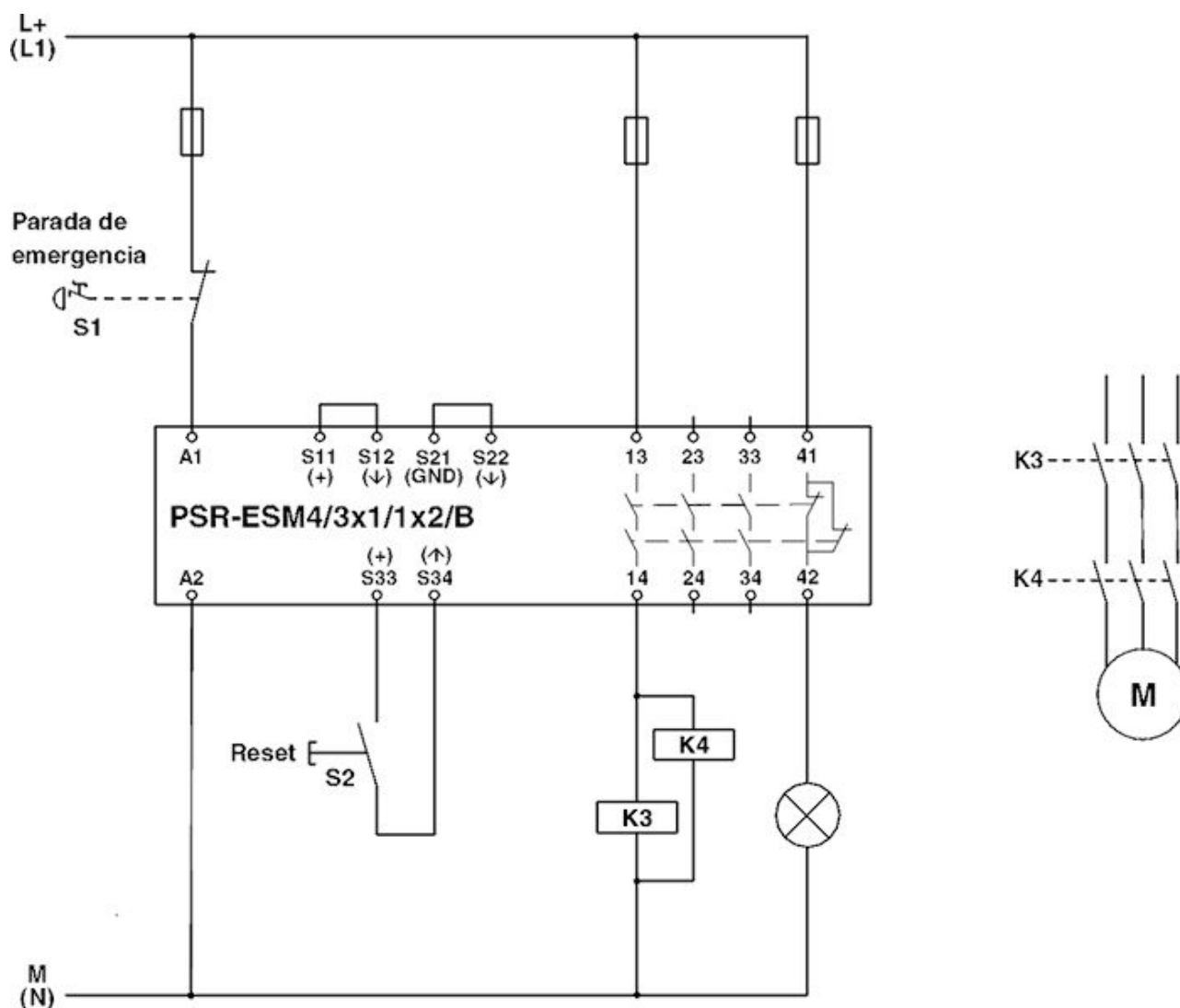
Diagrama eléctrico
