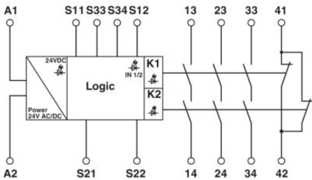
Diagrama eléctrico
