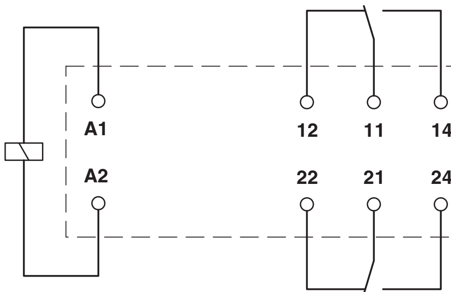
Diagrama eléctrico
