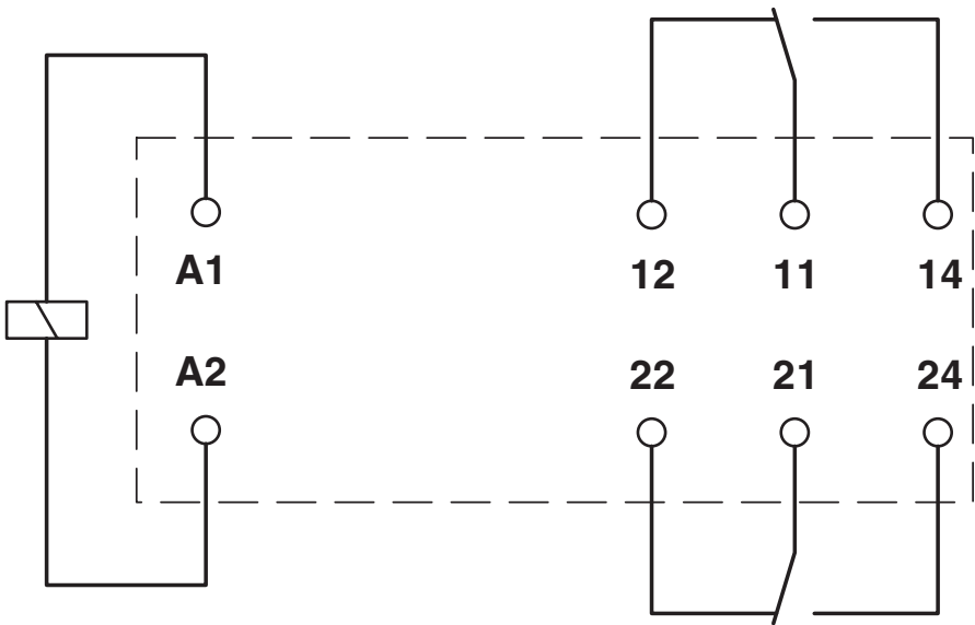
Diagrama eléctrico
