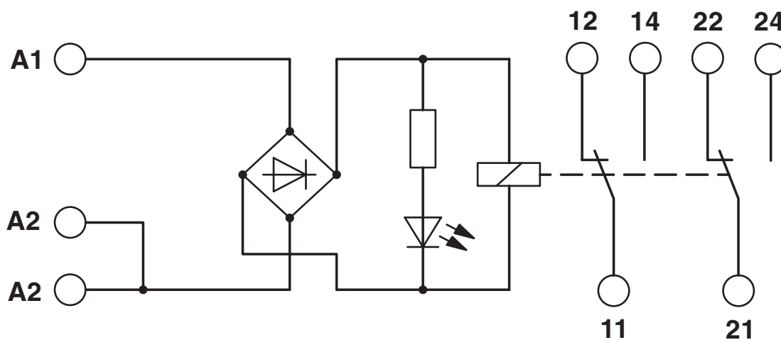
Diagrama eléctrico
