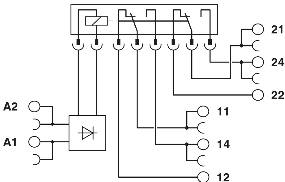
Diagrama eléctrico
