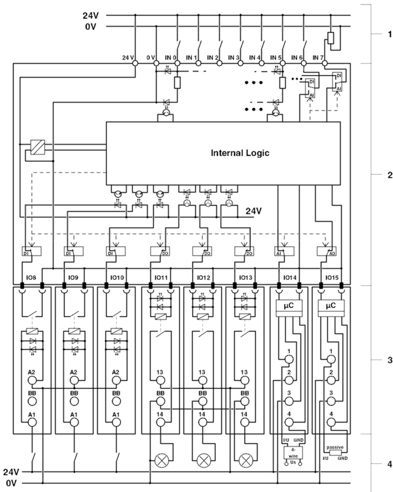
Diagrama eléctrico
