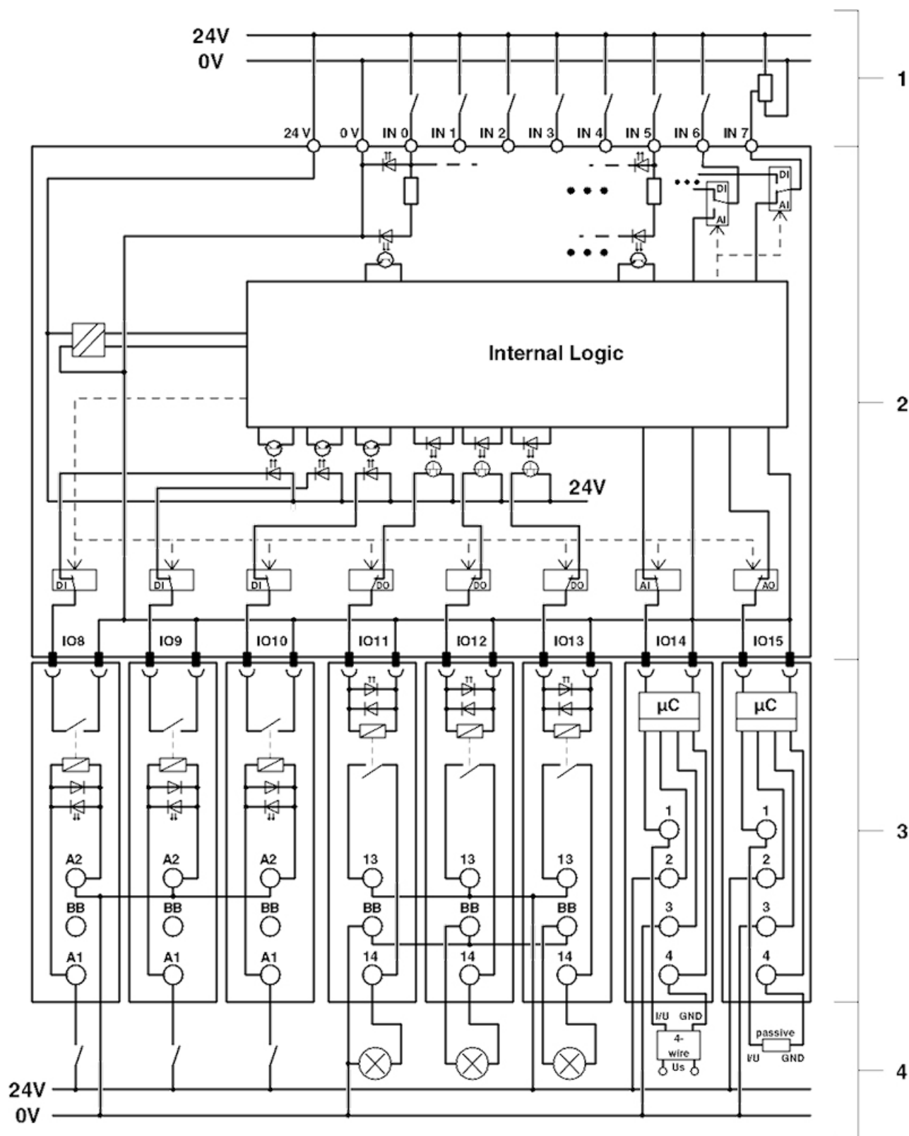
Diagrama eléctrico
