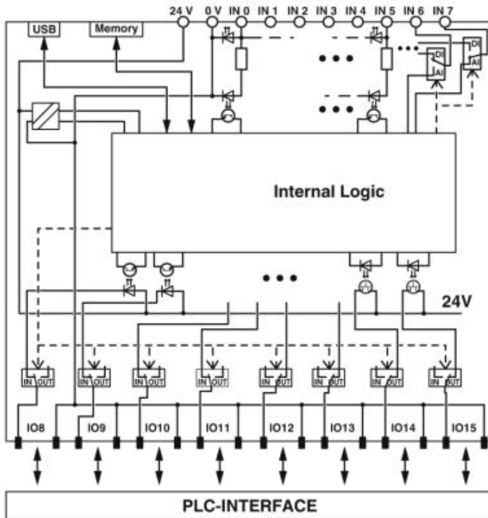
Diagrama eléctrico
