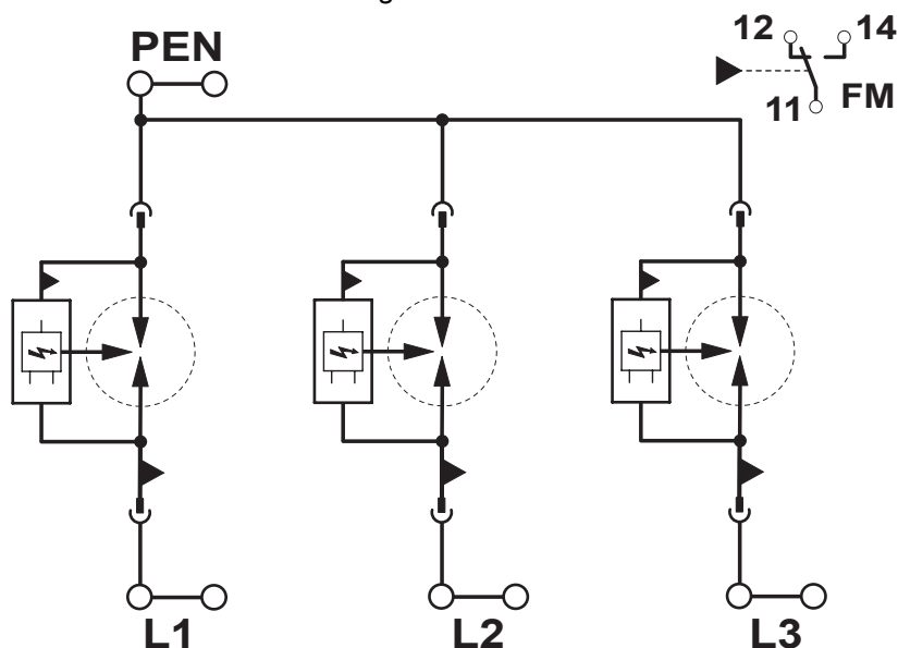
Diagrama eléctrico
