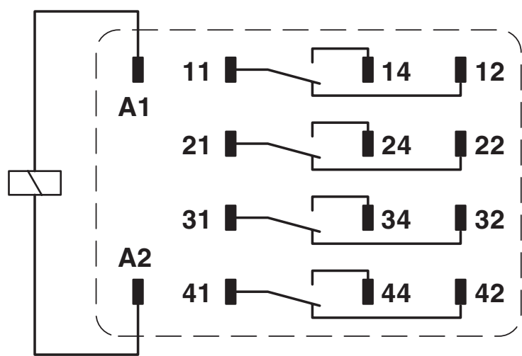
Diagrama eléctrico
