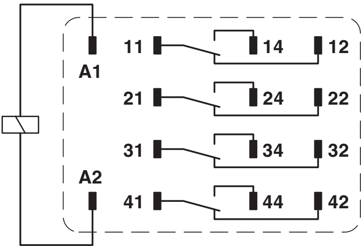
Diagrama eléctrico
