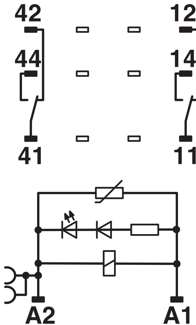
Diagrama eléctrico
