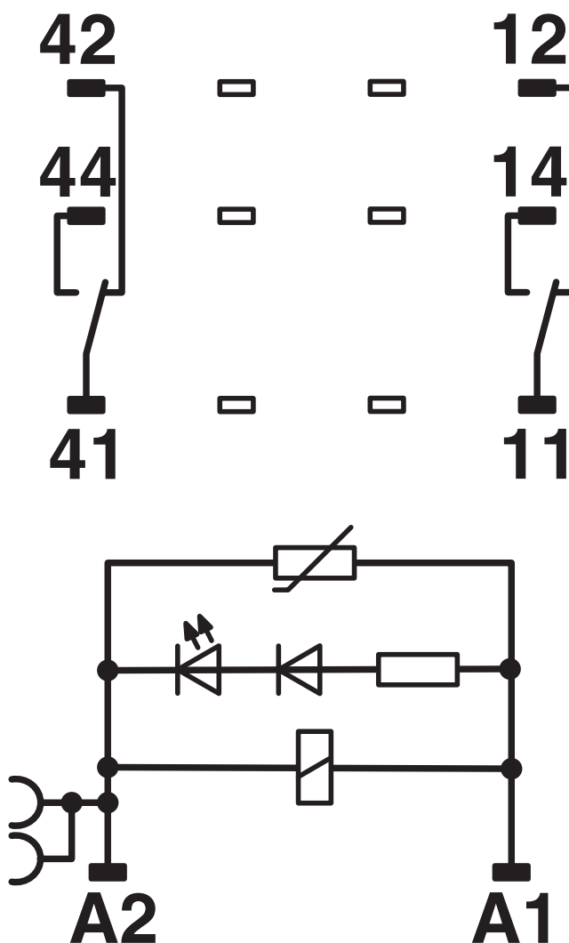
Diagrama eléctrico
