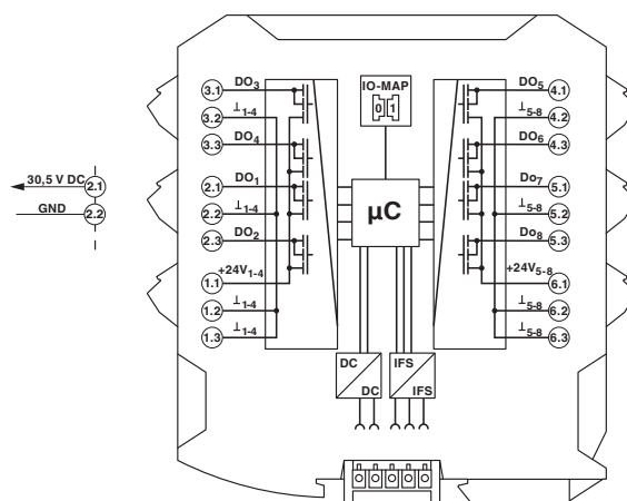
Diagrama eléctrico
