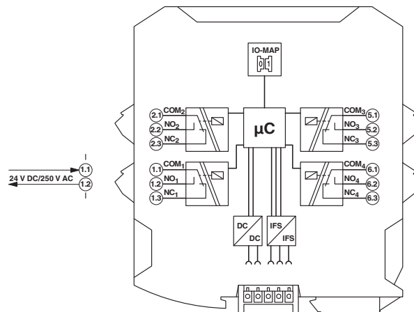
Diagrama eléctrico
