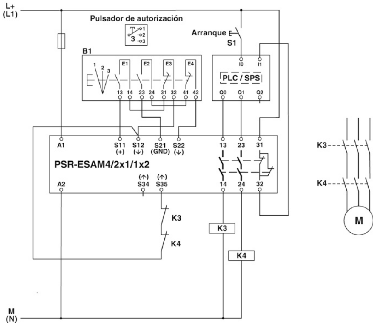
Diagrama eléctrico
