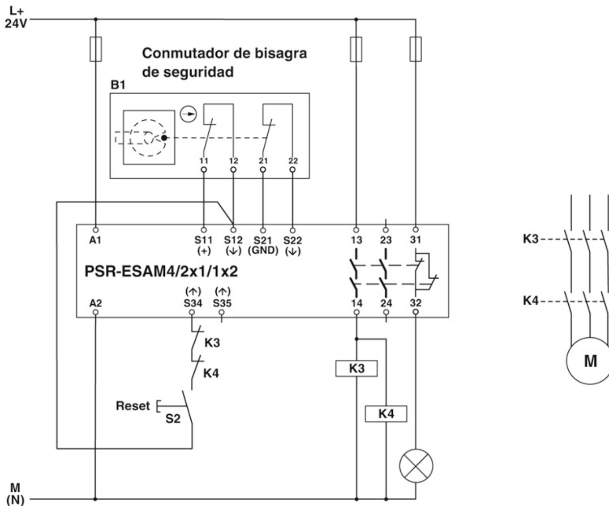
Diagrama eléctrico
