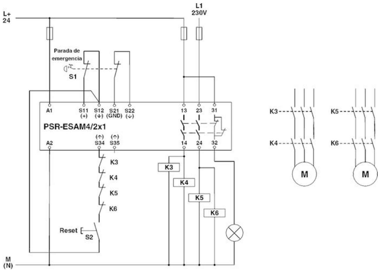
Diagrama eléctrico
