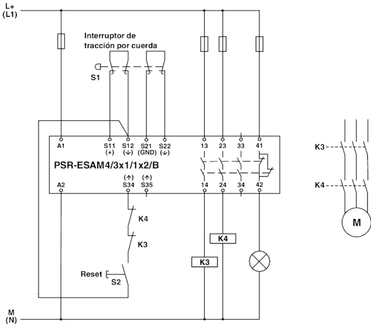
Diagrama eléctrico
