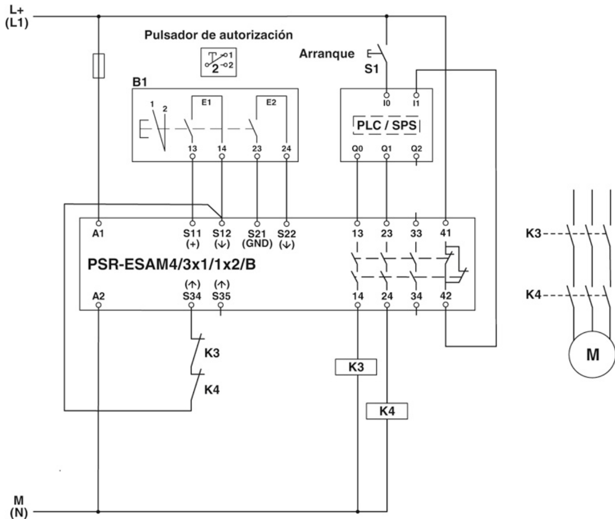
Diagrama eléctrico
