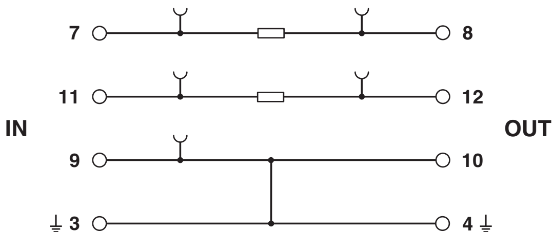
Diagrama eléctrico
