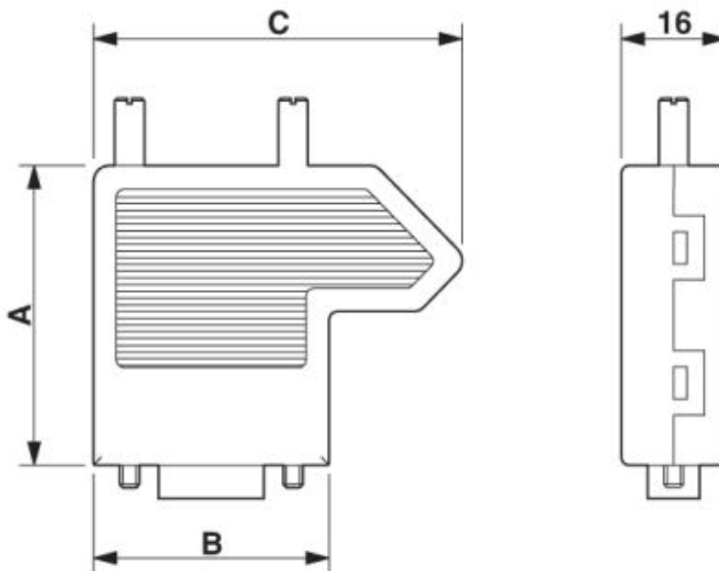
Plano esquemático
