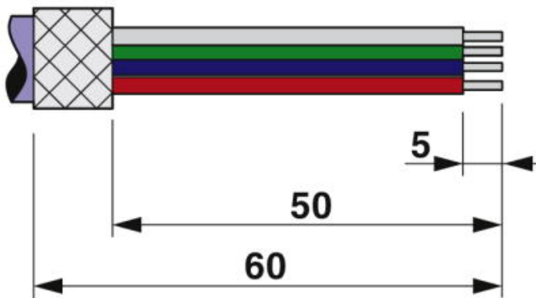
Plano esquemático
