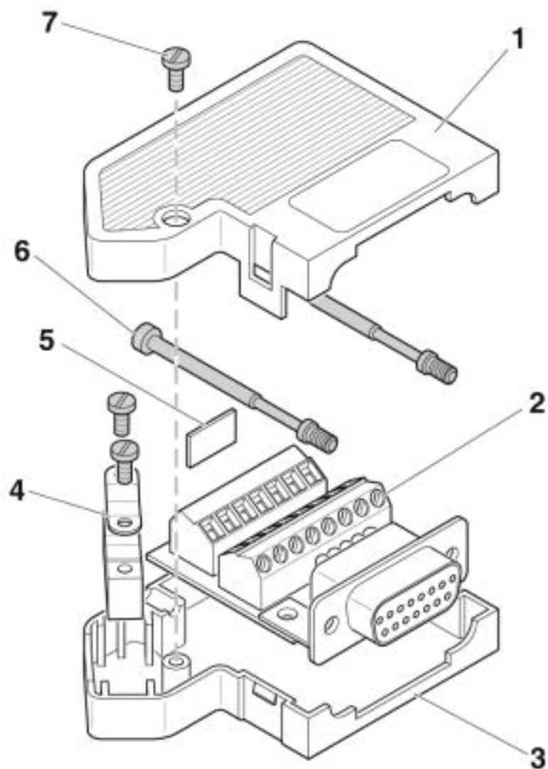
Plano esquemático
