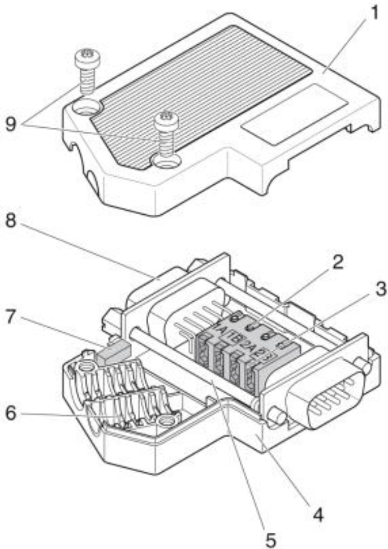
Plano esquemático
