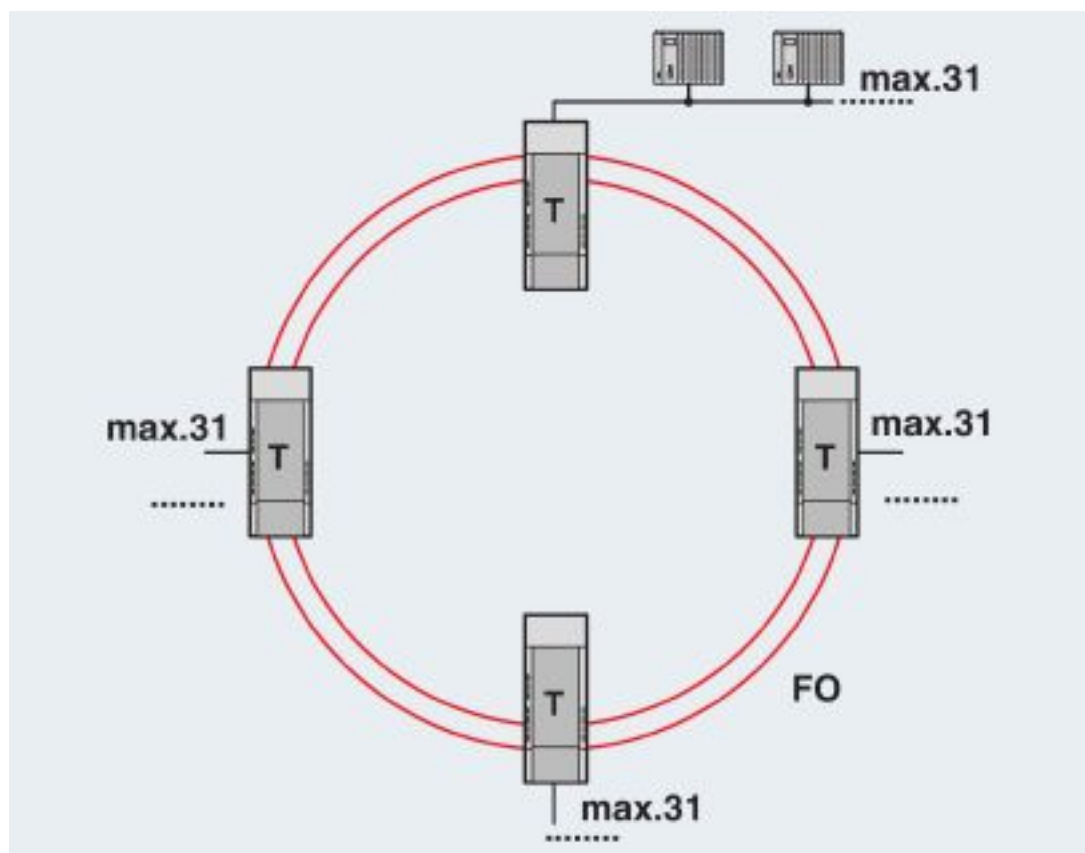
Anillo de fibra óptica redundante
