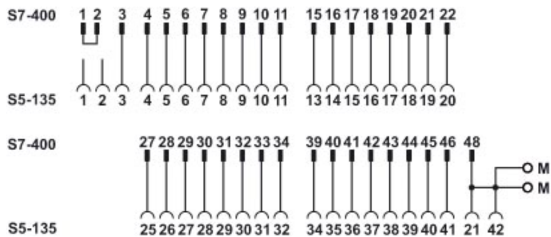
Esquema de conexiones FLKM S135/S400/SO121
