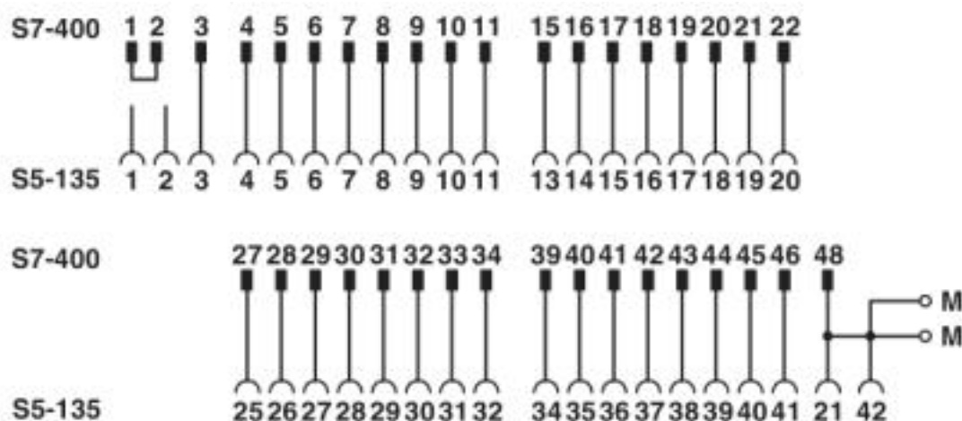
Esquema de conexiones FLKM S135/S400/SO121
