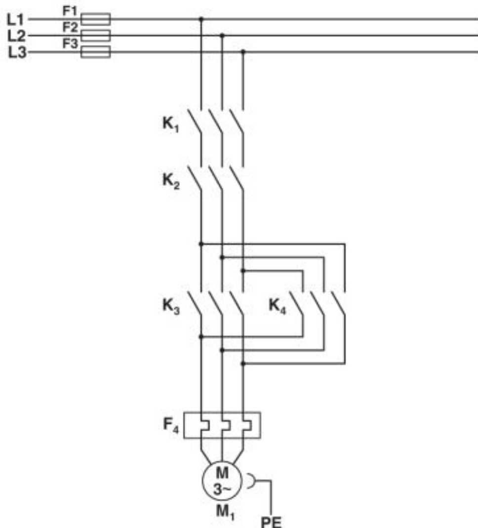
Diagrama eléctrico
