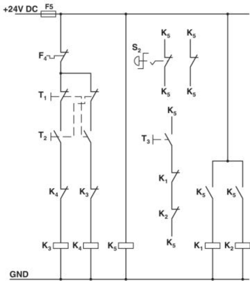
Diagrama eléctrico
