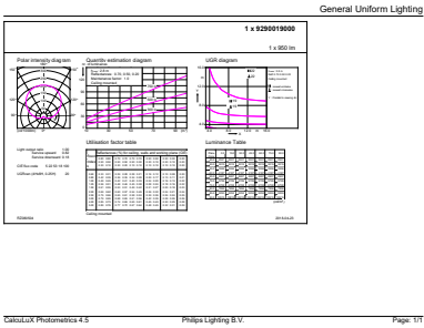
LEDbulb 9W A60 E27 765 FR
