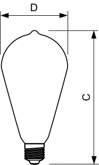
filament 7.5W-60W 806lm NAD 2700K E27ND
