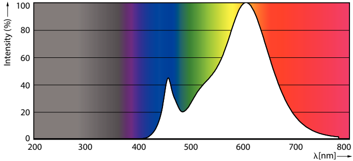
LEDCandle 5,5W B35 E14 827 FR
