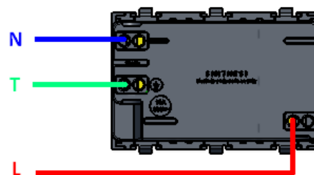
ESQUEMA CONEXION
