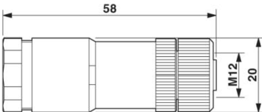
Conector hembra M12 x 1, recto
