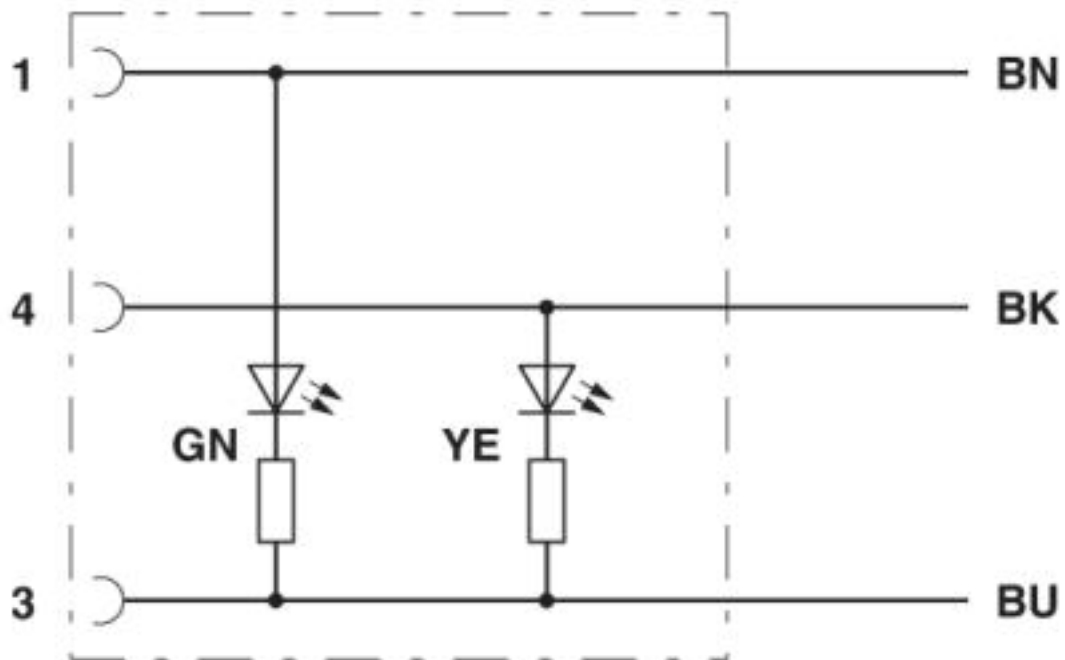
Diagrama eléctrico
