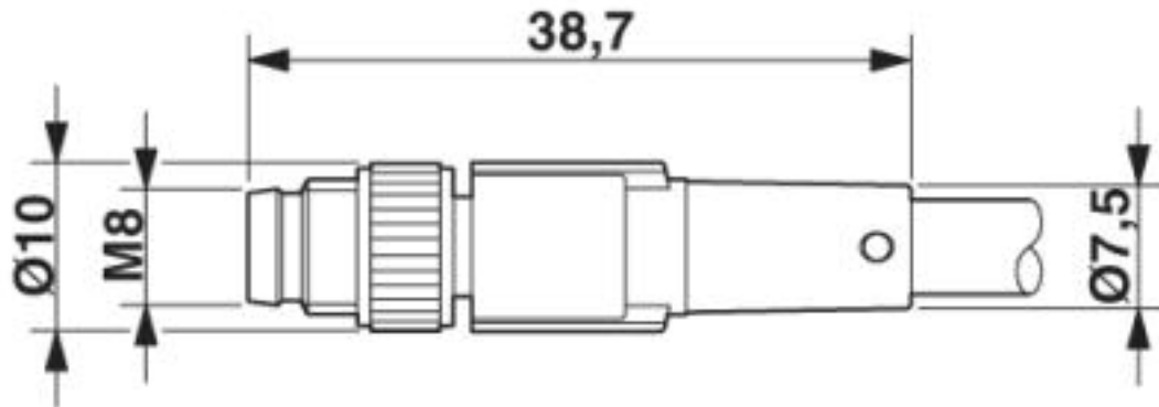
Conector macho M8 x 1, ejecución recta
