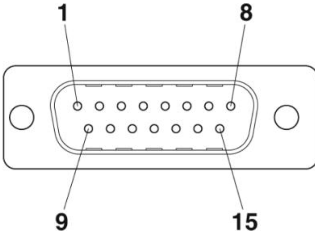
Plano esquemático
