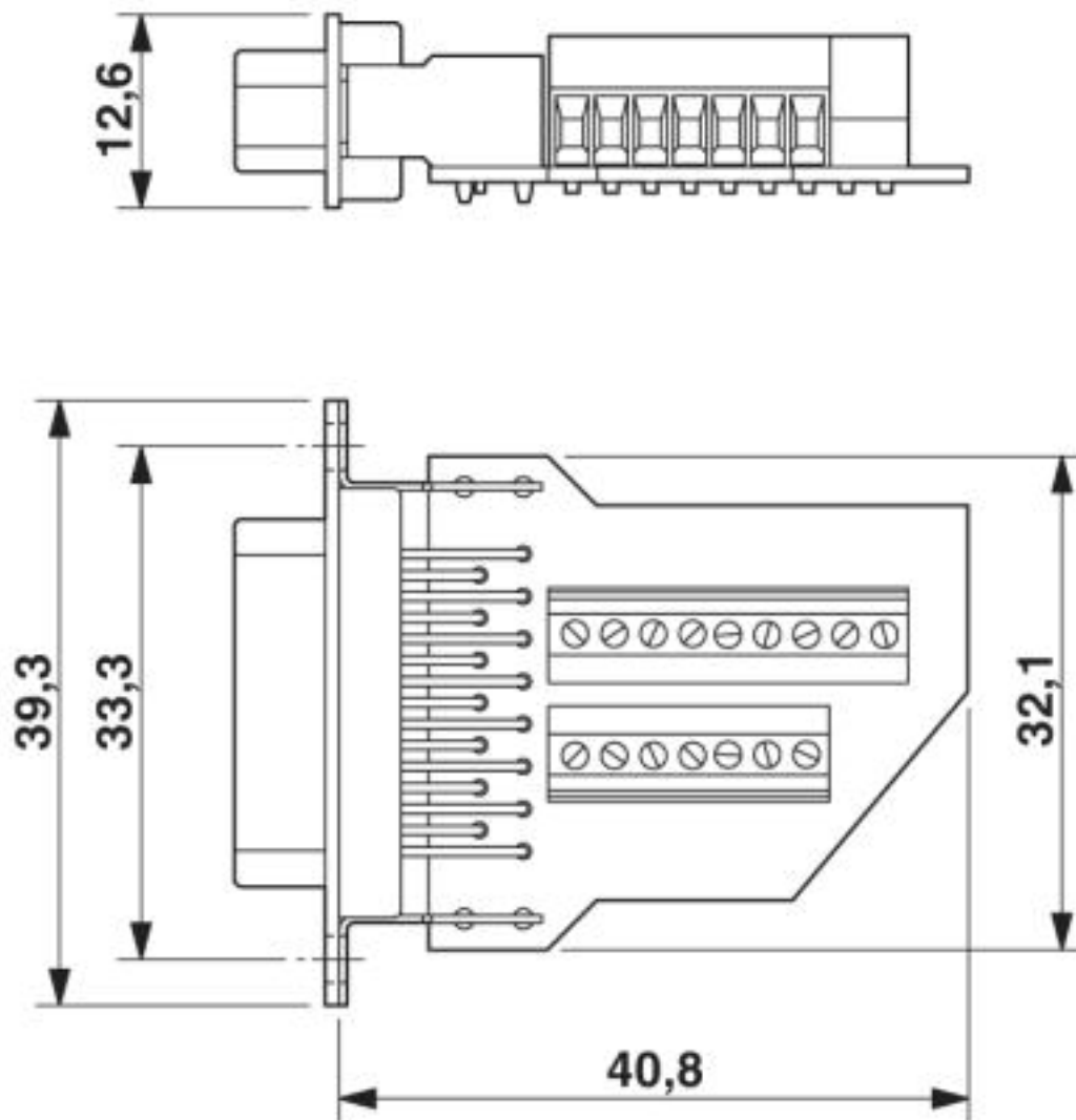
Inserto de contactos D-SUB
