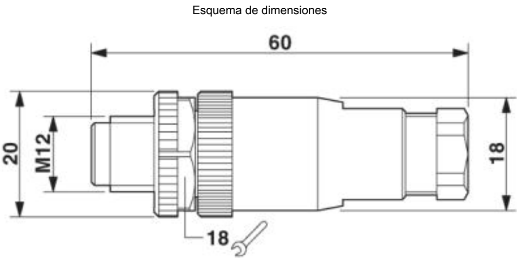
Conector macho M12 x 1, recto
