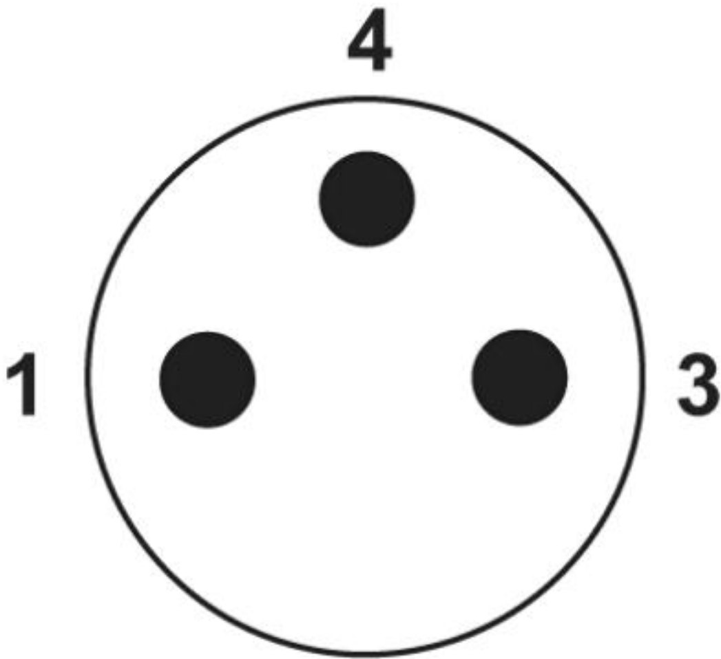
Esquema de polos del conector macho M8, de 3 polos
