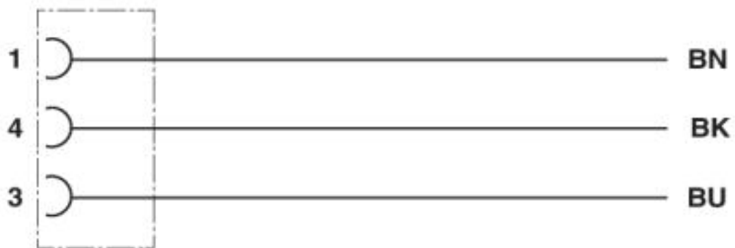
Diagrama eléctrico
