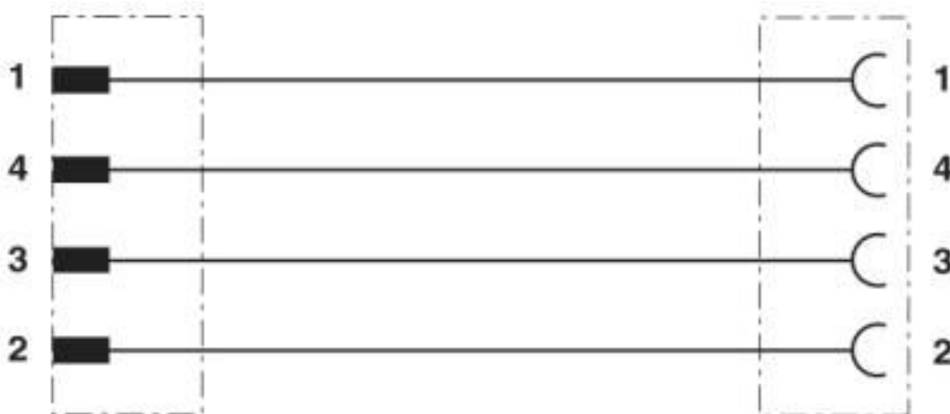
Diagrama eléctrico
